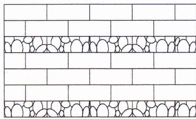
正面図
